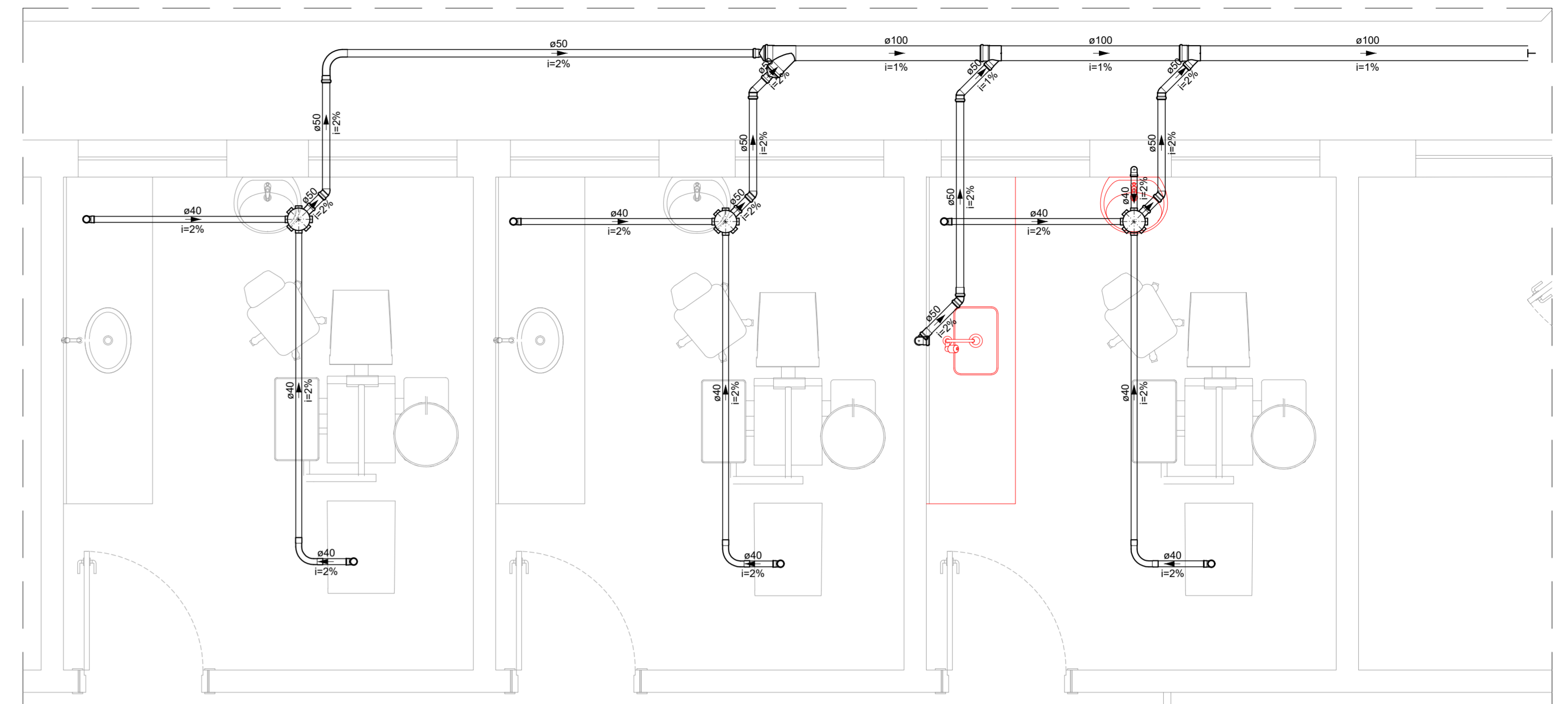
DET. SAN. - 1 Escala: 1:25
