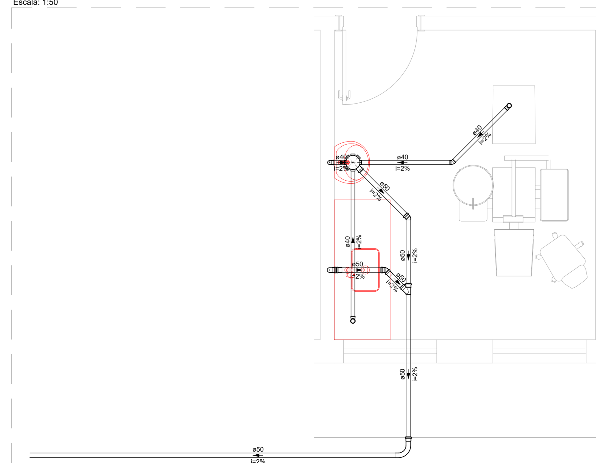
DET. SAN. - 2 Escala: 1:25
